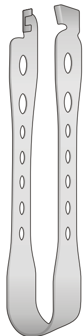
02-600-11 115 mm
