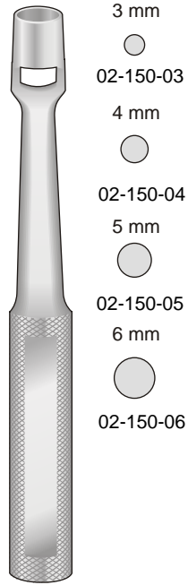
KEYES 02-150-10 100 mm
